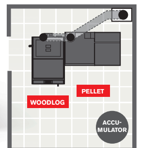
薪ボイラ（左） ペレットボイラ（右）
